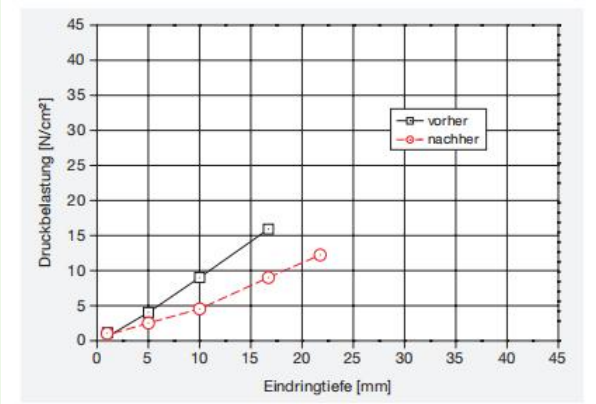
Bild 2: Verformbarkeit in Abhängigkeit vom Auflagedruck
